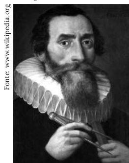
Figura 5: Kepler
