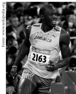
Figura 13: Usain Bolt.
