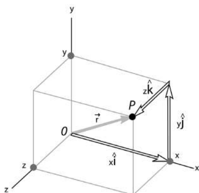
Figura 13: Vetor Posição
