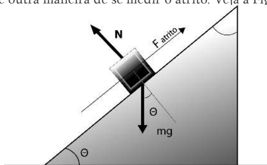
Figura 20: Outro modo de medir o coeficiente de atrito
