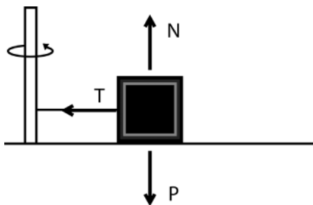
Figura 24: Diagrama de forças
