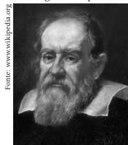
Figura 6: Galileu
