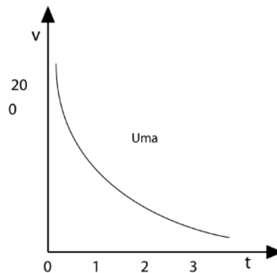
Figura 12 – Gráfico da hipérbole
