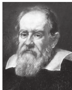
Figura 2: Galileu Galilei
