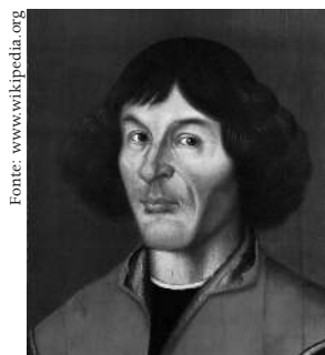
Figura 3: Copérnico
