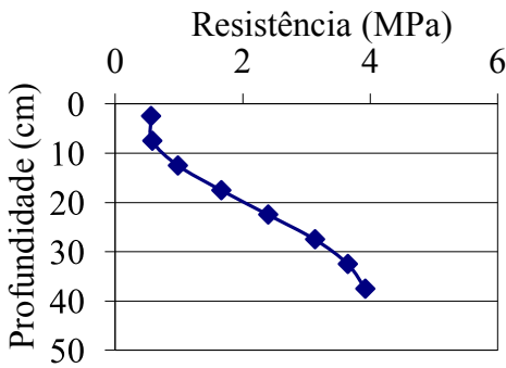
Figura 1. Resistência do solo a penetração (RSP) antes da implantação do experimento. Sítio do Sol, Seropédica, RJ. Abril de 2018.
