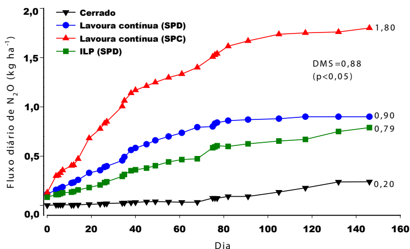
Figura 13. Fluxo diário de óxido nitroso quantificado durante o ciclo do sorgo safrinha em sucessão à soja em experimento de longa duração na Embrapa Cerrados, Planaltina-DF.
