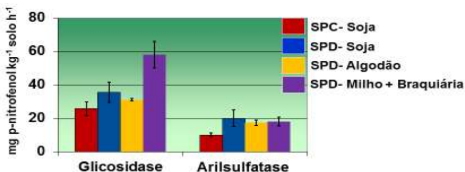
Figura 7. Atividade enzimática (mg de p -nitrofenol kg de solo -1 h -1 ) de um Neossolo Quartzarênico (0-10 cm) sob diferentes sistemas de manejo na Fazenda Xanxerê (Correntina, BA). Teores médios de MOS de 6 g kg -1 .
