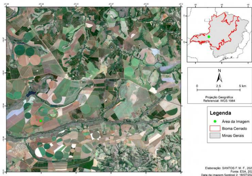
Figura 9. Imagem de satélite de uma área representativa da região III. Notar a presença abundante de pivôs de irrigação, os amplos interflúvios e o uso intensivo do solo. Fonte imagem: ESA, 2020. Elaborado: pelos autores.
