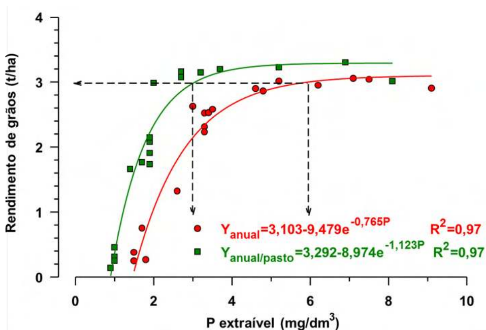
Figura 12. Efeito de sistemas de cultivo com (verde) e sem (vermelho) braquiária na relação entre o fósforo extraível por Mehlich-1 na camada de 0-20cm de profundidade e a produtividade da soja no 13º cultivo. Fonte: Sousa et al. (1997).
