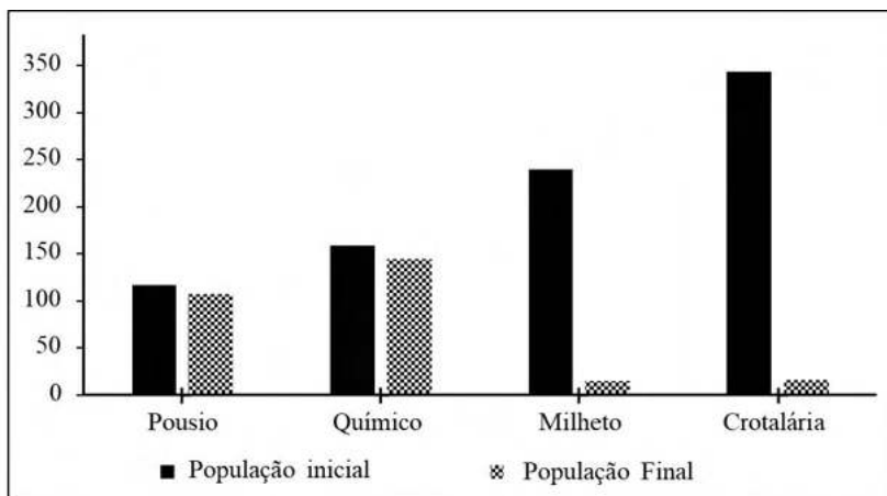
Figura 4. População inicial e final de Meloidogyne incognita em amostras de solo e raízes, em Uberaba-MG. Fonte: Ferreira et al. (2021).
