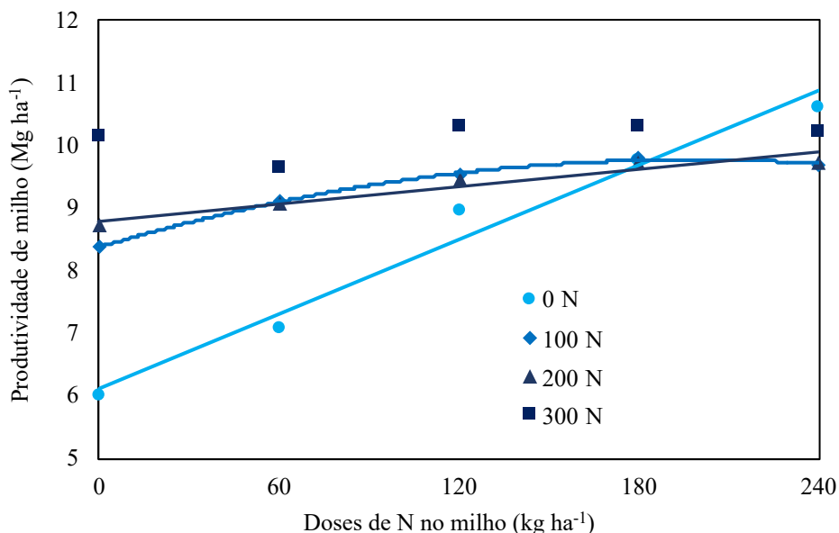
Figura 4. Produtividade de milho em um sistema integrado de produção agropecuária após diferentes doses de N aplicadas na pastagem de aveia preta + azevém em antecedência em Guarapuava, Paraná. Fonte: adaptado de Assmann et al. (2003).
