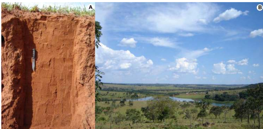
Figura 15. Latossolo Vermelho-Amarelo Distrófico argissólico, textura média (A); Paisagem típica das áreas com ocorrência do Grupo Bauru no Triângulo Mineiro. Originalmente predominavam a fitofisionomia de cerrado em Latossolos em sua maioria vermelhos (B). Fotos: Guilherme R. Corrêa.
