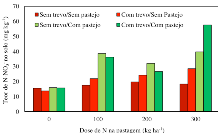
Figura 3. Teores de nitrogênio na forma de nitrato (N-NO 3 - ) no solo de acordo com doses de N aplicadas no inverno, em áreas com ou sem a presença de trevo e com ou sem a presença de pastejo, em Guarapuava, Paraná. Fonte: adaptado de Assmann et al. (2003).
