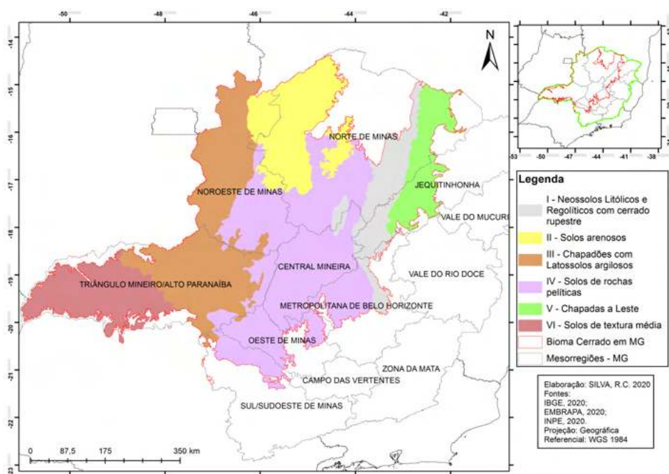
Figura 2. Domínios com padrões de potencialidades e fragilidades de solos ocupados originalmente pela vegetação do Cerrado.
