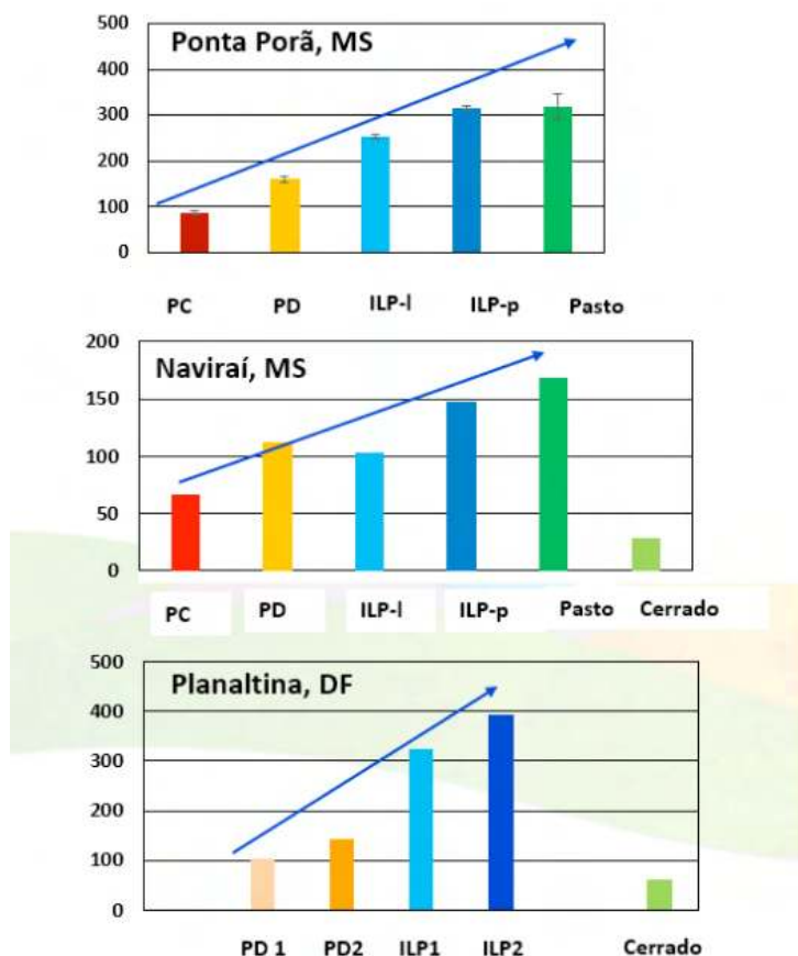
Figura 6. Atividade da arilsulfatase nos experimentos de ILP da Embrapa Cerrados (Planaltina, DF; responsável: Dr. Lourival Vilela) e Embrapa Agropecuária Oeste (Naviraí e Ponta Porã, MS; responsáveis: Dr. Júlio C. Salton e Dr. a Michely Tomazi).
