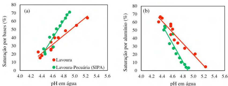
Figura 2. Relação entre pH (em água) e saturação por bases (a) e saturação por alumínio (b) do solo em área com 17 anos de sistema plantio direto e histórico de cultivo agrícola, onde o sistema integrado de produção agropecuária (SIPA) (soja-bovinos de corte) havia sido adotado há nove anos, em São Miguel das Missões, Rio Grande do Sul.
