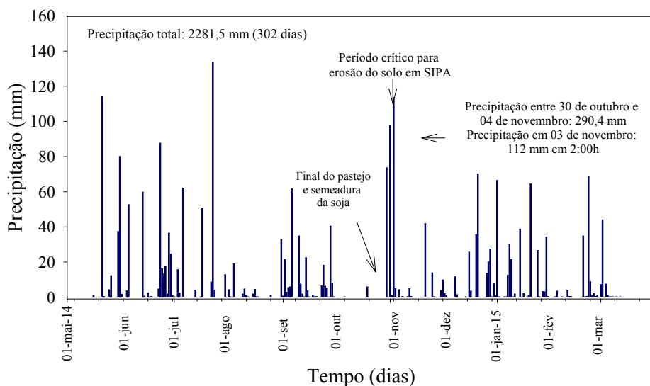
Figura 4. Precipitação pluviométrica em uma área experimental em sistemas integrados de produção agropecuária durante o cultivo de soja e ciclo de pastejo em São Miguel das Missões, Rio Grande do Sul.
