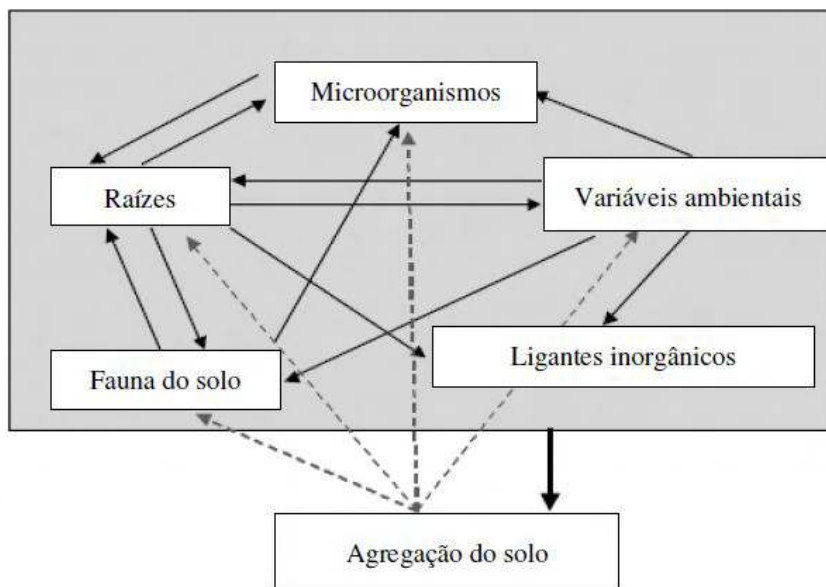
Figura 3. Esquema demonstrando a multiplicidade de interações entre os cinco principais fatores que influenciam a formação e estabilização dos agregados do solo.
