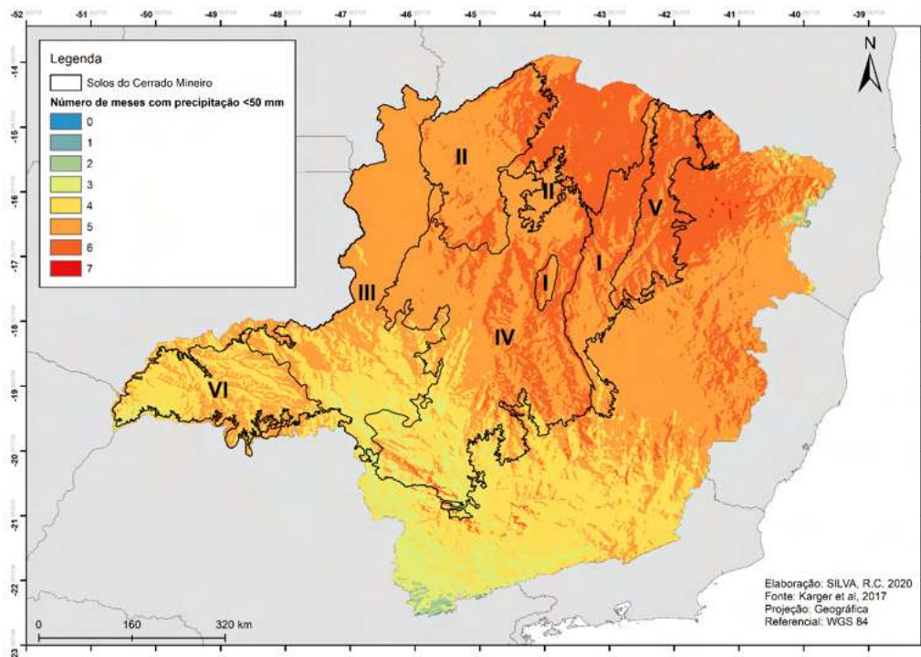
Figura 17. Mapa do número de meses com precipitação inferior a 50 mm. Fonte: Karger et al. (2017). Elaborado pelos autores.
