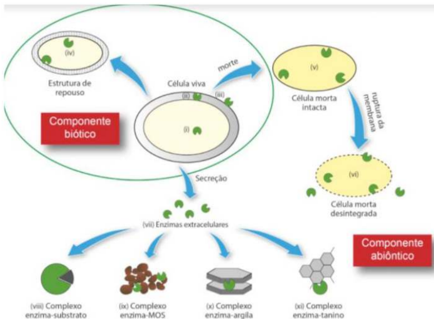
Figura 3. Esquema ilustrativo da localização das enzimas nos compartimentos solo. Fonte: Adaptado de Wallenstein e Burns (2011).
