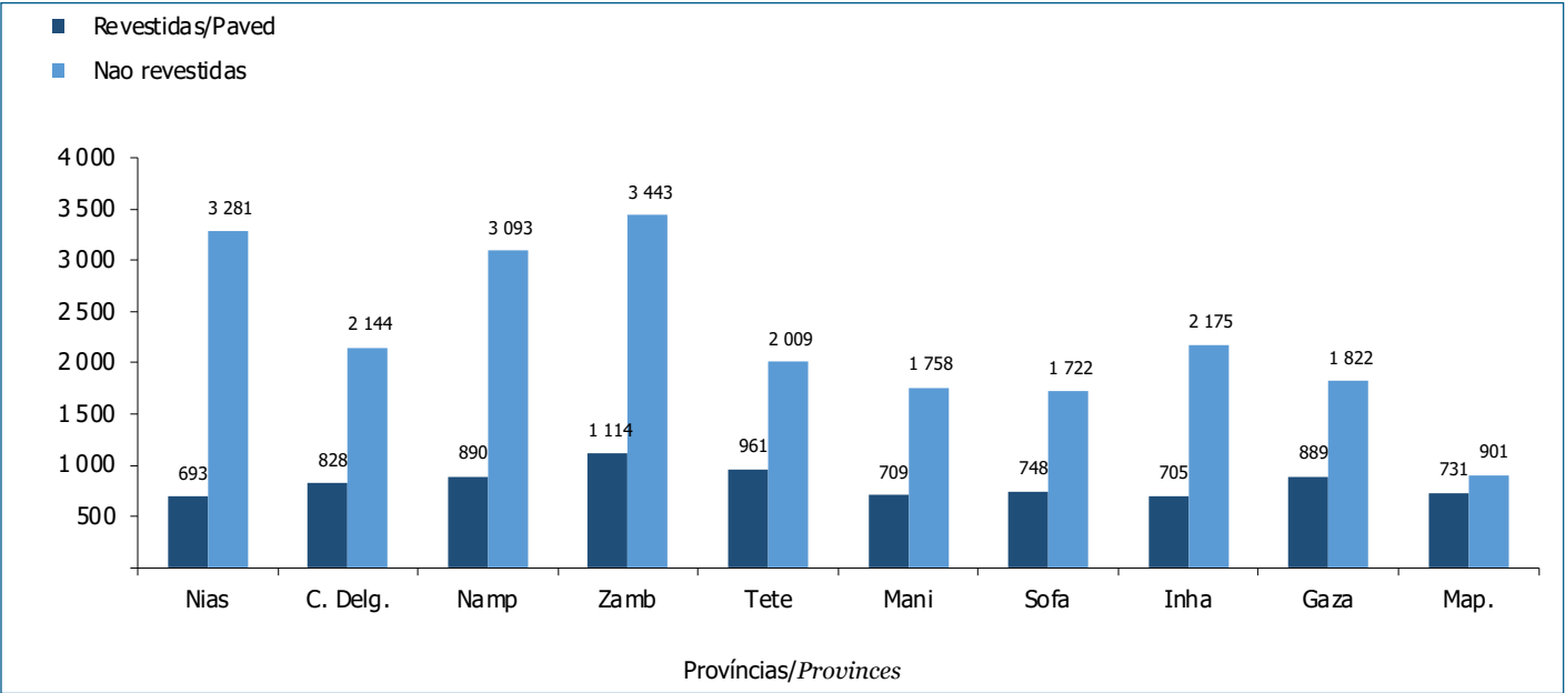
Gráfico 3.9.3.1 Extensão da rede de estradas por tipo de superfície segundo província. Moçambique, 2023
